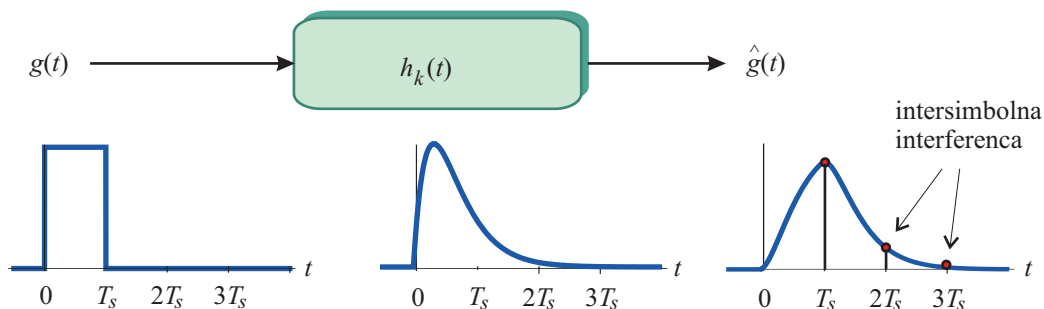
Slika 7.3 – Popačenje impulza pri prenosu. Impulz se raztegne po časovni osi. Pri sprejemu bi tak impulz vzorčili pri njegovi maksimalni vrednosti. Problem je, da se razteza tudi v čas, ko bi vzorčili naslednji impulz in pokvari njegov vzorec. Pride do medsebojnega vpliva med oddanimi simboli ali intersimbolne interference
