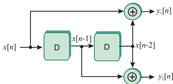
Slika 11.11 – Konvolucijski kodirnik z s kodnim razmerjem k = 1/2 . Kodirnik je pravzaprav končni avtomat. Izhodni biti so odvisni od stanja kodirnika, to je simbolov shranjenih v D celicah in vhodnega bita. Ob vsakem urinem taktu, se spremeni stanje kodirnika glede na vhodni bit.
