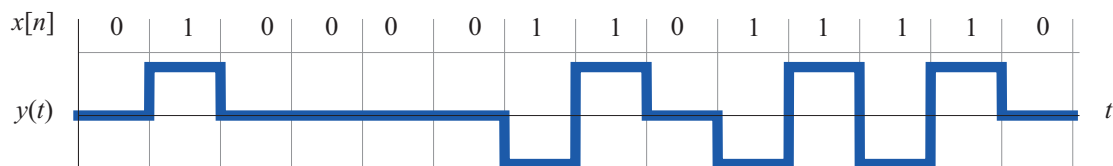
Slika 11.7 – Pri AMI kodi se predznak simbola 1 izmenjuje, zato je sprotna digitalna vsota omejena. Pri dolгих zaporedjih samih 0, pa lahko še vedno pride do izgube sinhronizacije.
