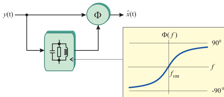
Slika 4.18 – Demodulator sukanjem faze in faznim detektorjem. Fazo vhodnega signala najprej zasučemo z nihajnim krogom, ki ima v območju okrog centralne frekvence dokaj linearno fazno karakteristiko. S faznim detektorjem nato primerjamo fazo originalnega in fazno zasukanega signala. Ker je fazni zasuk odvisen od trenutne frekvence frekvenčno moduliranega signala, je signal na izhodu enak modulacijskemu signalu.
