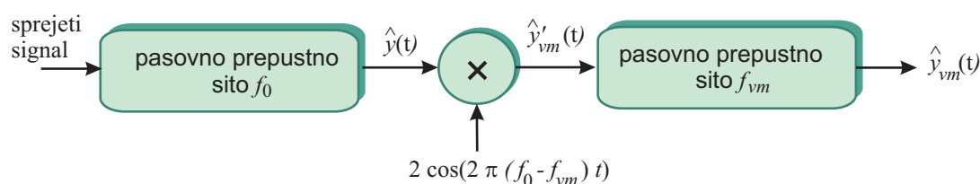
Slika 4.6 – Načelna vezava mešalnika navzdol. S sitom pred mešalnikom izločimo zrcalno frekvenco, s sitom po mešalniku pa izločimo sosednje frekvence (sosedne kanale).
